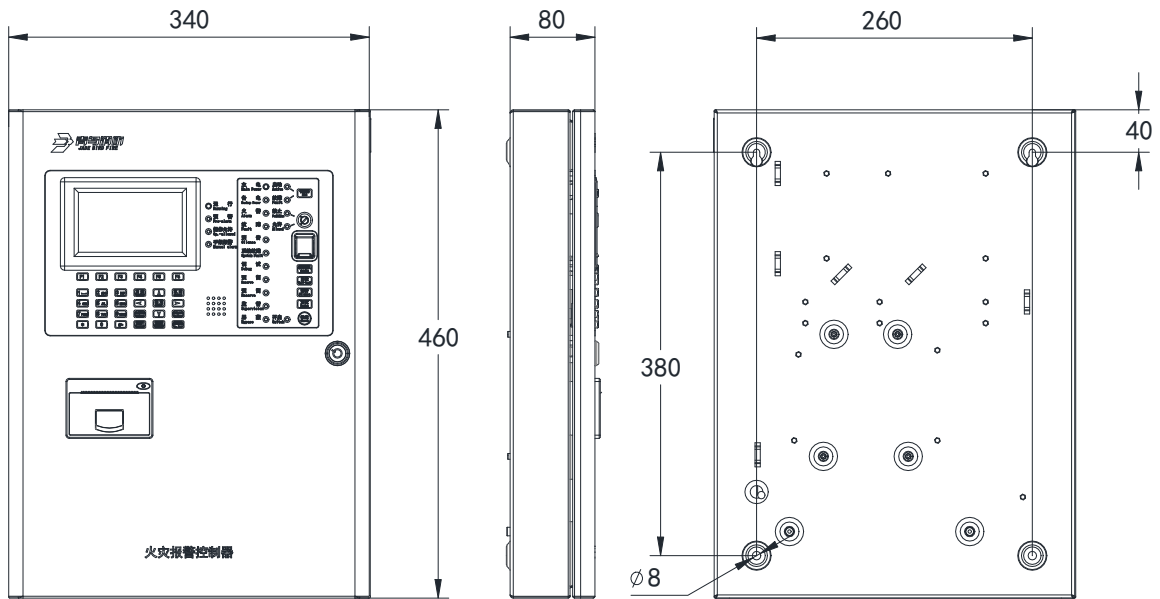
控制器尺寸图
