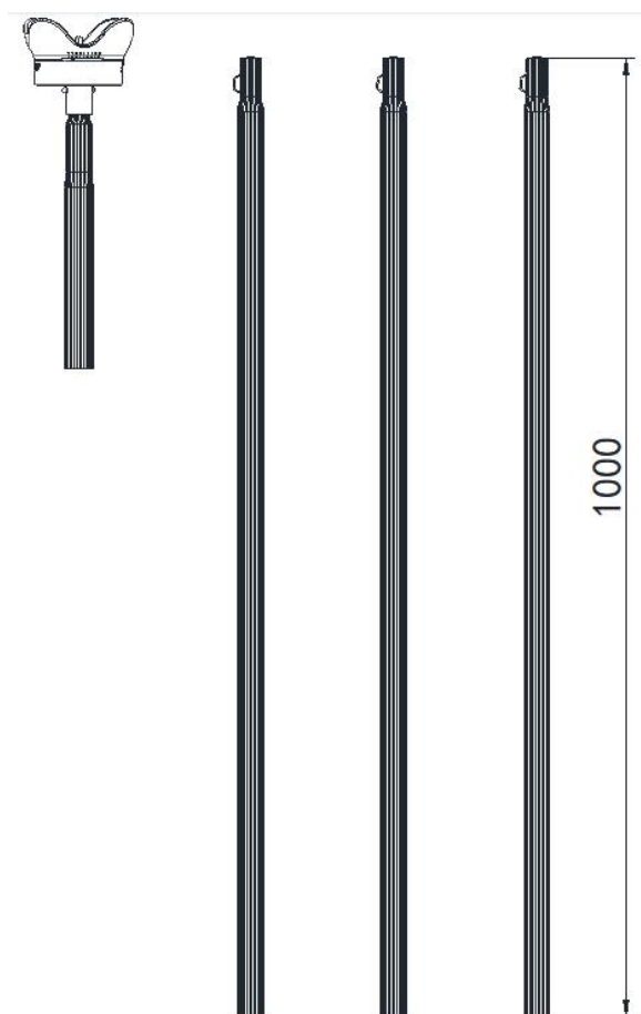
图 2 外形尺寸图
