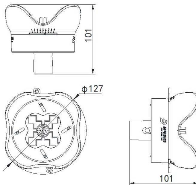
图 1 外形尺寸图
